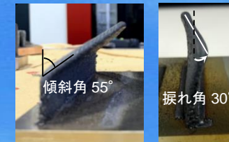
傾斜角と捩れ角を持つ積層体
